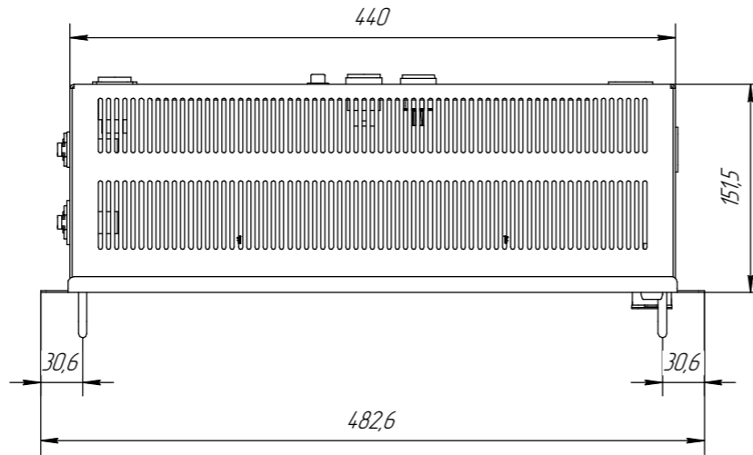
Вид сверху
